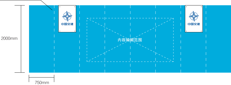
彩钢瓦式围挡色彩使用宽博蓝
