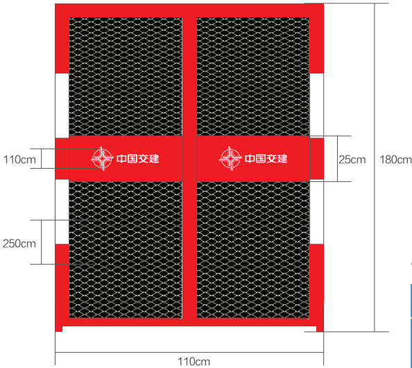
层站防护门
